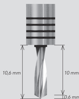
Esempio di fresa \varnothing 2 \times lungh. 10 mm
