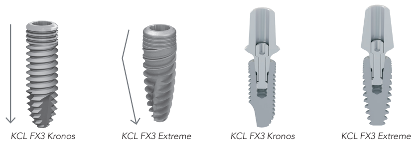
Sezione impianto e pilastro
